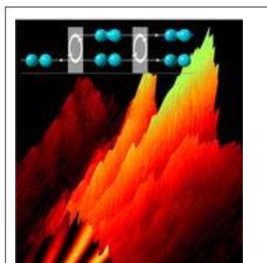
Bild: Interferometer für Rydberg-Moleküle: Durch einen Laserpuls (im Schema grau) werden Paare von Rubidium-Atomen in einen Überlagerungszustand zwischen freien Atomen und gebundenem Molekül gebracht. Mit einem zweiten Puls kann die unterschiedliche zeitliche Entwicklung der beiden Zustände auf die Anzahl der Moleküle überführt werden, welche dann gemessen werden (durch Farbe und Höhe der Fläche dargestellt). Universität Stuttgart
